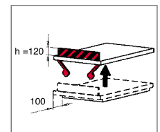
Abrollsicherung
